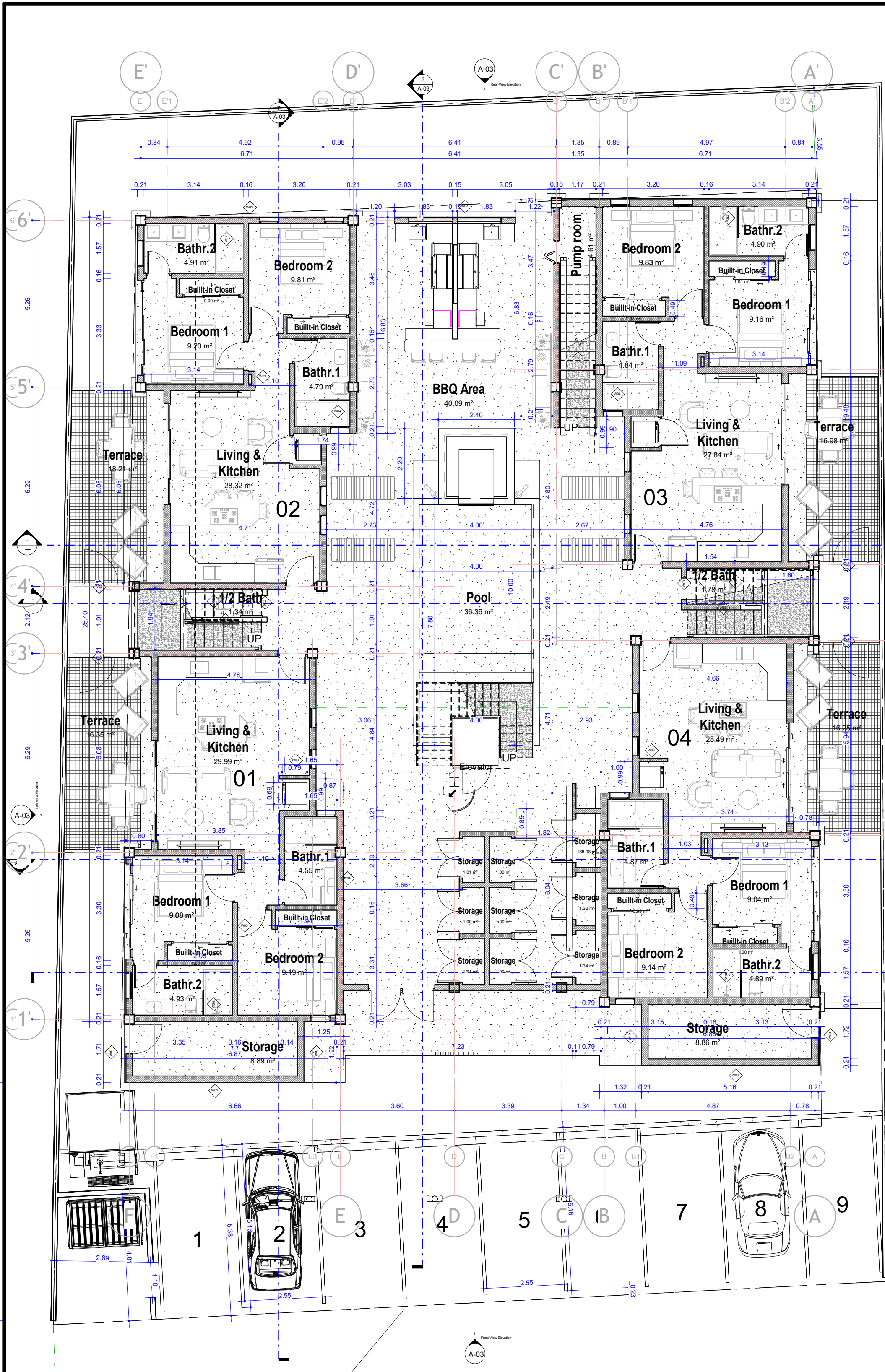
1 Floorplan 1 : 100
